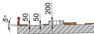
剖面 A-A
