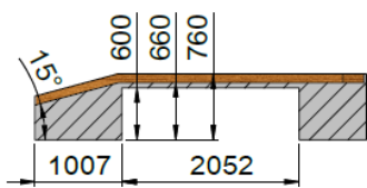
剖面 B-B
